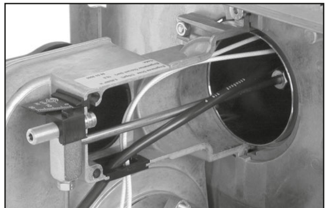
Afbeelding 27 — Demontage van de verstuur afdek plaat
