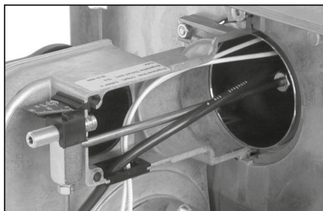
Figure 27 — Démontage du boîtier de raccordement du gicleur
