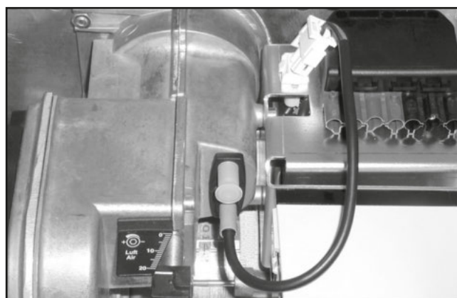
Figure 29 — Prise de raccordement de la cellule photo-électrique
