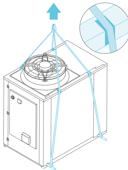
Levage avec système d'élingues
