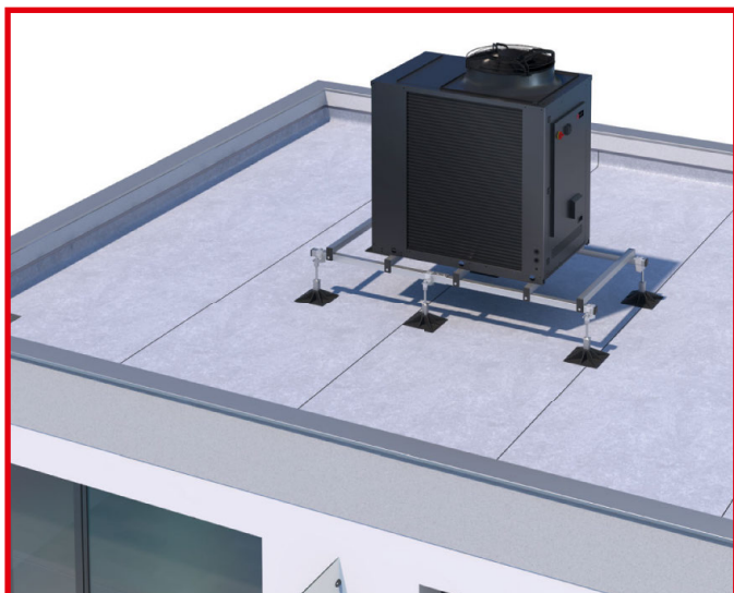
installation en toiture terrasse
