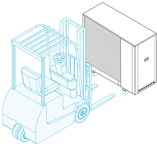
Levage avec chariot élévateur
