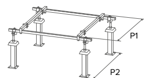
Support sous-étanchéité châssis M
