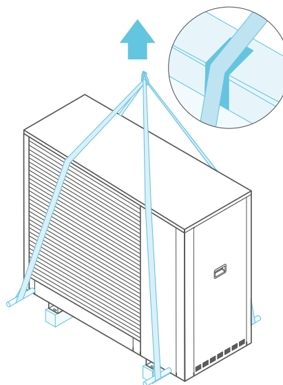
Levage avec sangles/chaînes
