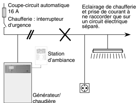
Schéma 3 : Conduite électrique dans la chaufferie
