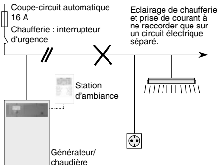
Schéma 3 : Conduite électrique dans la chaufferie
