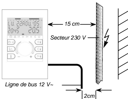
Schéma 1 : Ecart minimum pour installation électrique
