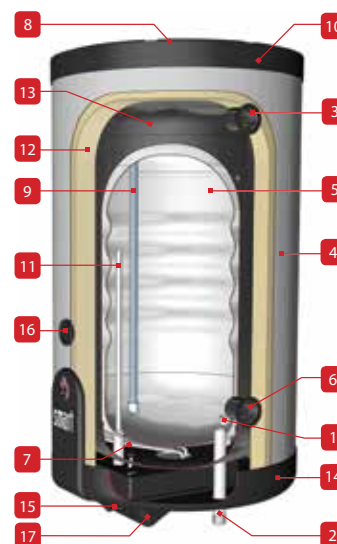
Smart EW - verticale wandbevestiging met de sanitaire aansluitingen verplicht naar onder gericht. Primaire kring steeds vullen.
