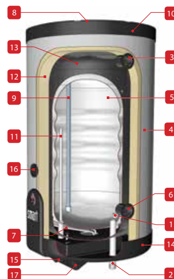
Smart EW - Installation murale verticale raccordement sanitaire vers le bas. Le côté primaire doit toujours être rempli.
