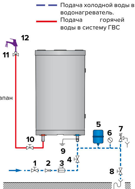
Вертикальный монтаж
