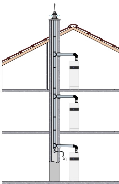
Cascade met een schouwaansluiting configuratie C43
