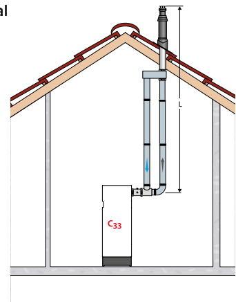
Parallel schouwkanaal
