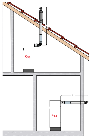
Concentrisch schouwkanaal
