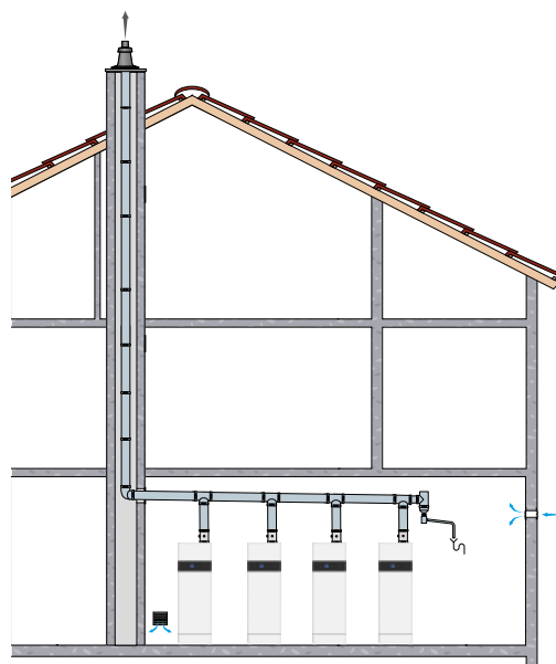
Cascade met een schouwaansluiting configuratie B23
