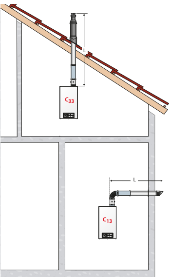
Conexión concéntrica
