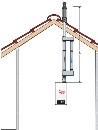
Conexión paralela
