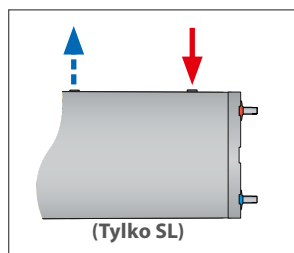
(Tylko SL) Instalacja pozioma - pozycja wisząca
