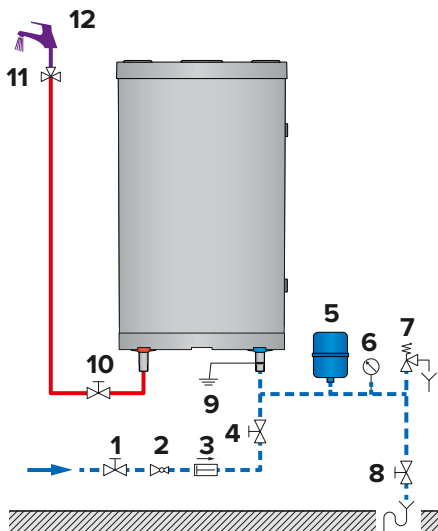
Installazione verticale
