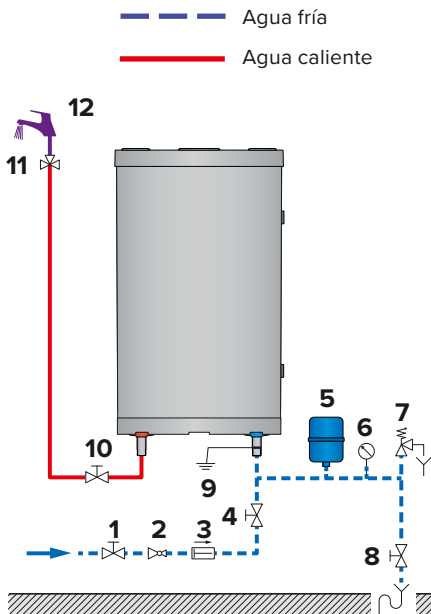
Montaje vertical
