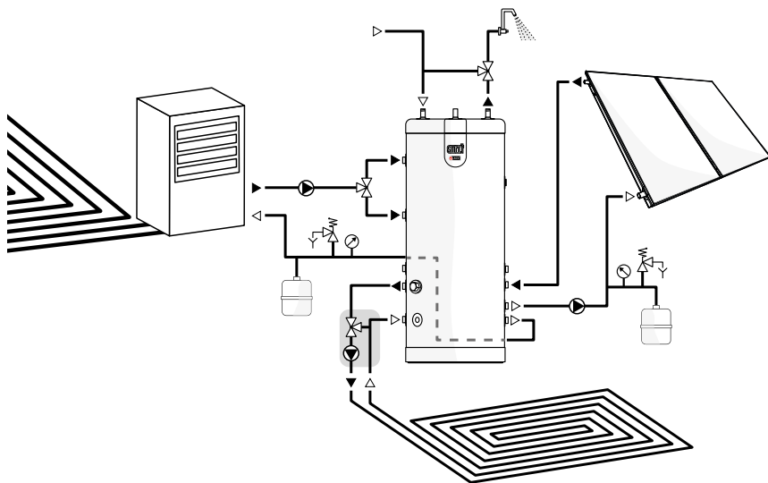
Smart ME in Kombination mit Wärmepumpe, Solaranlage und Fußbodenheizung.
