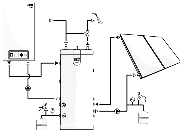
Smart ME in Kombination mit Heiztherme und Solaranlage.
