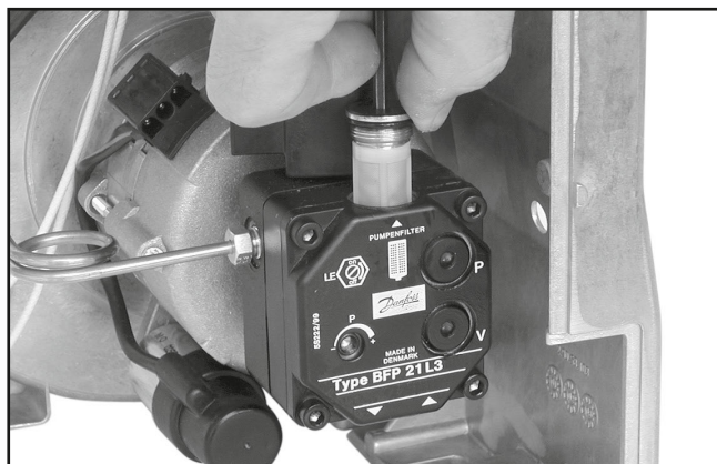
Figure 25 — Démontage du filtre à fioul
