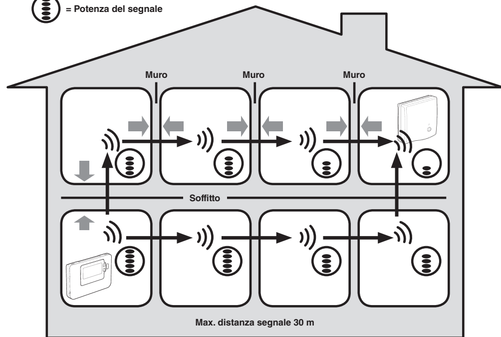
Tipico esempio di perdita di segnale nella struttura di un edificio
