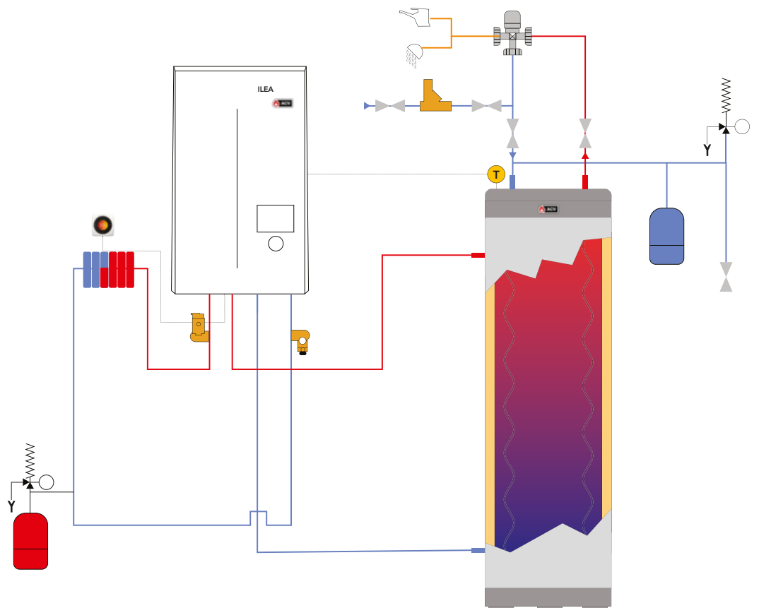
ILEA SOLO + OPSLAGTANK VOOR SANITAIR WARM WATER PRODUCTIE
