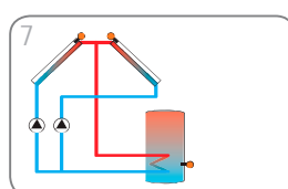
Zonne-energiesysteem met oost- / westdak (pagina 14)
