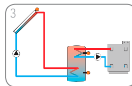
Zonne-energiesysteem met 1 boiler en naverwarming (pagina 10)
