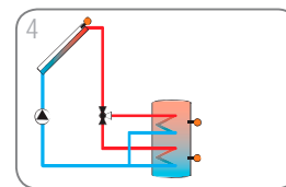
Zonne-energiesysteem met 1 boiler en 3-wegklep voor boilerlagenvulling (pagina 11)
