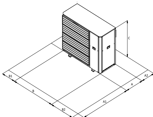
figure 8 - Dégagements minimums d'installation autour de l'unité extérieure
