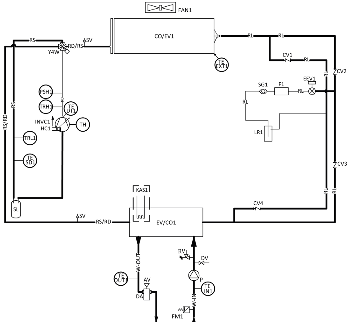
figure 12 - Schéma des organes de la PAC
